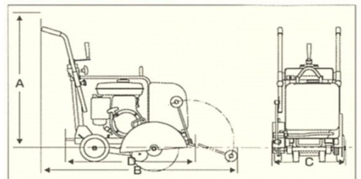
寸法図 & 寸法表 単位:mm
